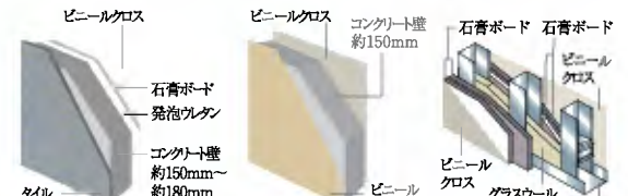
外壁構造図
