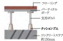
二重床構造図
