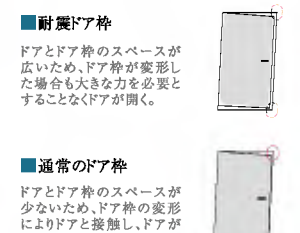
耐震ドア枠
